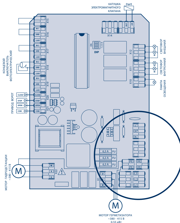
Рис. 5.2.1. Вид А. Подключение источника питания
