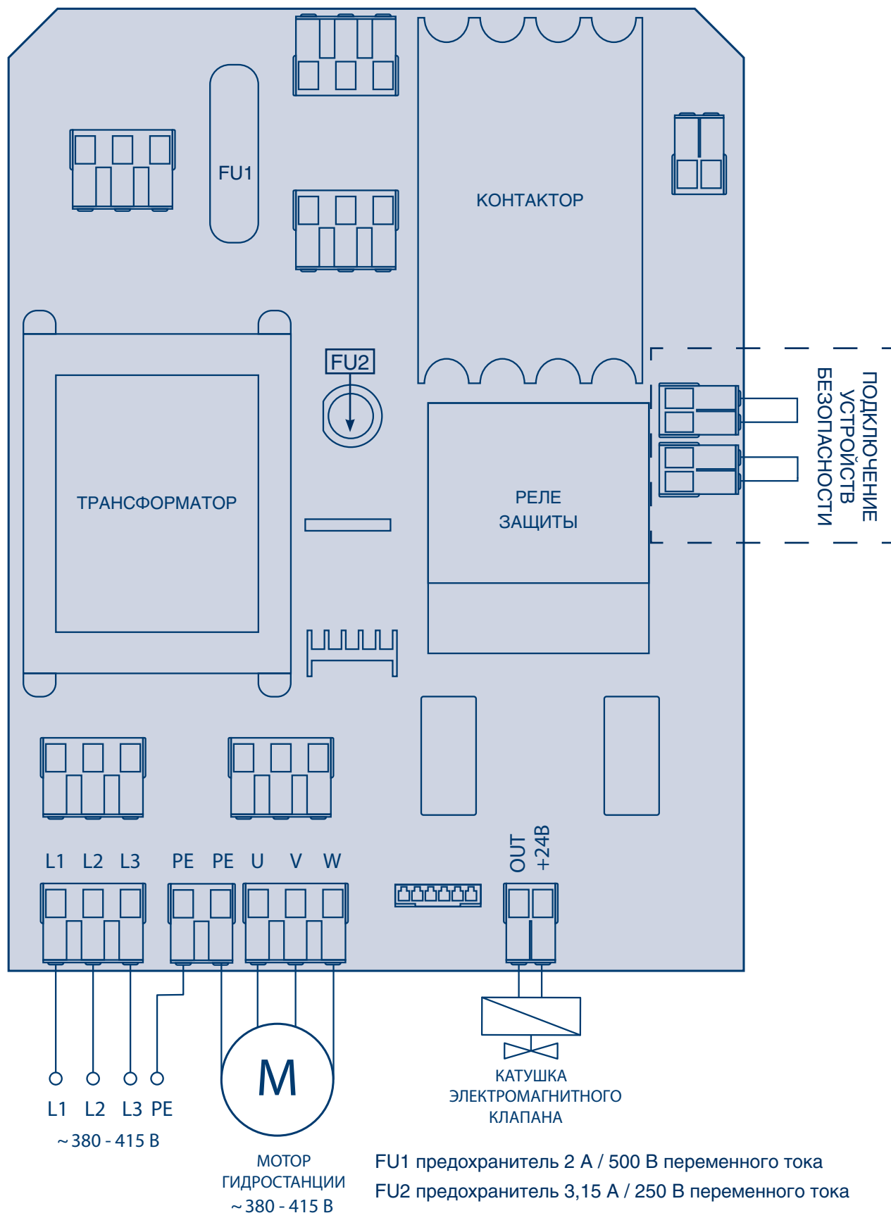
Рис. 5.1. Общая схема электрических подключений
