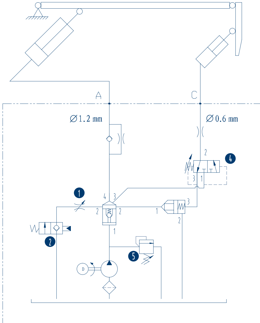
Рис. 4.5. Гидросхема
