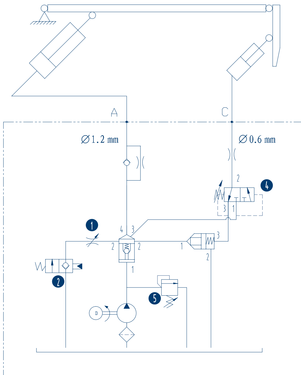
Рис. 3.4. Гидросхема
