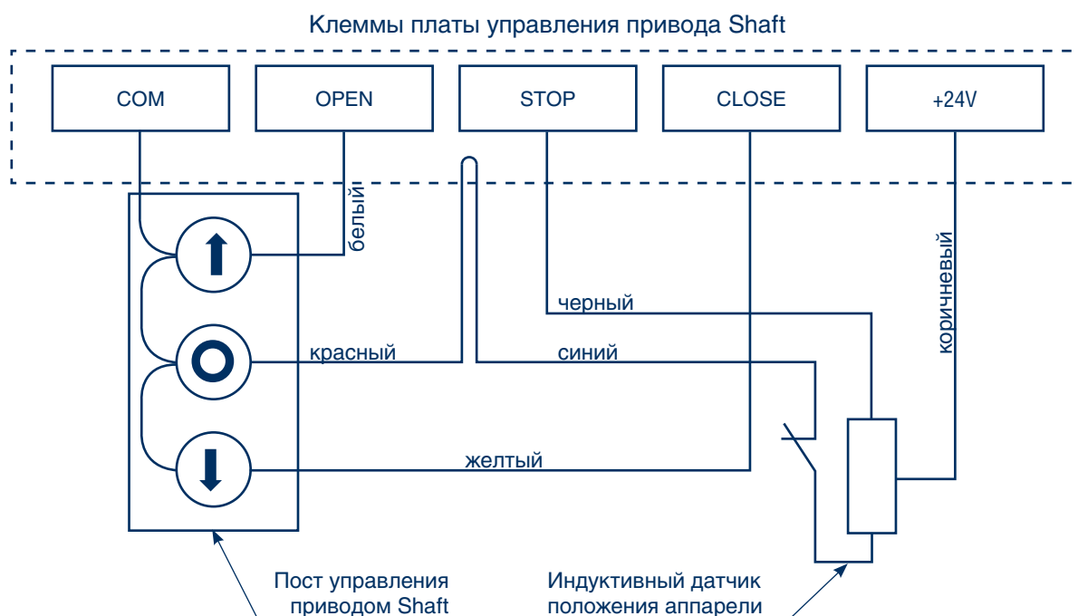
Рис. 5.2. Схема подключения индуктивного датчика положения аппарата*
