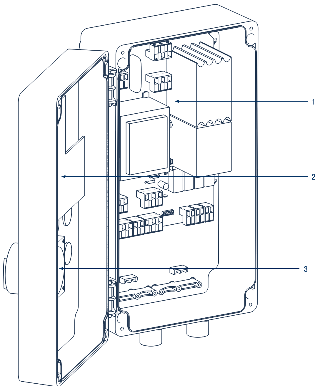
Рис. 1. Конструкция блока управления
