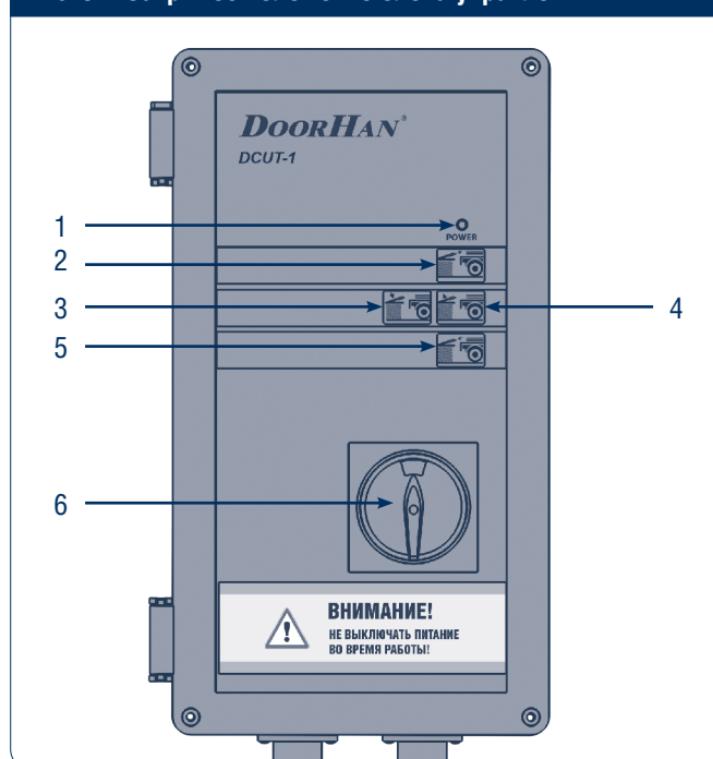
Рис. 3.1. Закрытое положение блока управления
