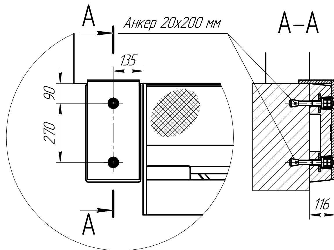
Бампер резиновый 450x250x100 со стальной рабочей накладкой 16мм (артикул BRSP(16)465x250x165 ) Комплектуется анкерными болтами 20x200 мм, в кол-ве 2 шт.
