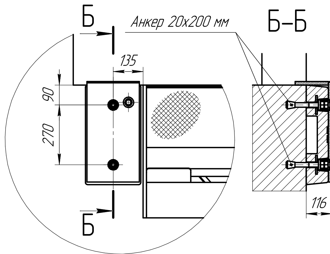
Бампер резиновый 450x250x100 со стальной раб. накладкой 16мм и датчиком парковки (артикул BRSP(16)465x250x165S ) Комплектуется анкерными болтами 20x200 мм, в кол-ве 2 шт.
